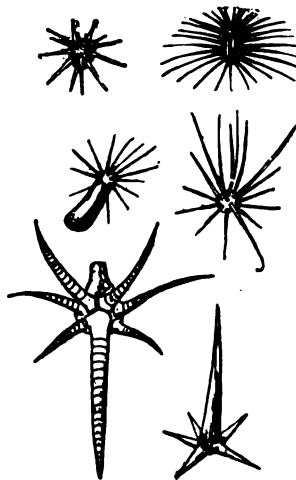
716. Cactus spines.
