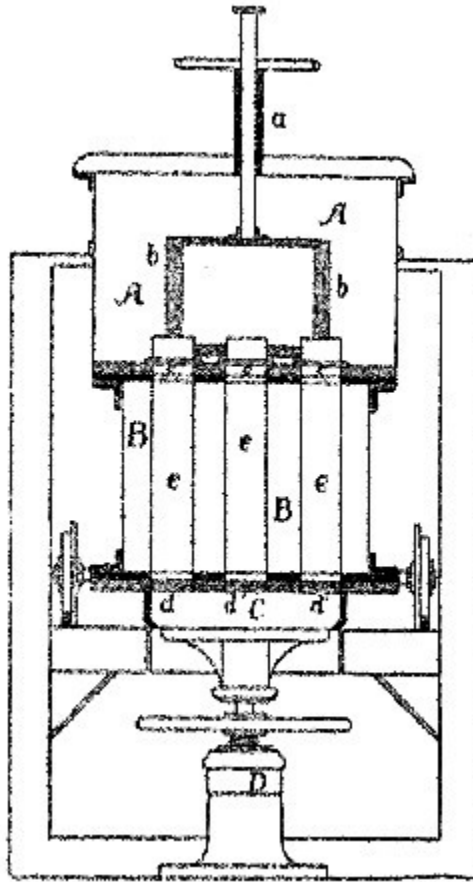
Fig. 19.—Leimdoerfer cooler.
