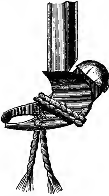
Fig. 514.—Half turn.
