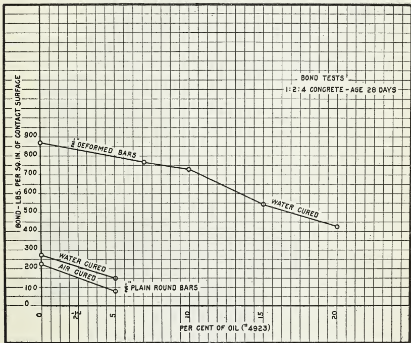
FIG. 7.—Bond tests.
