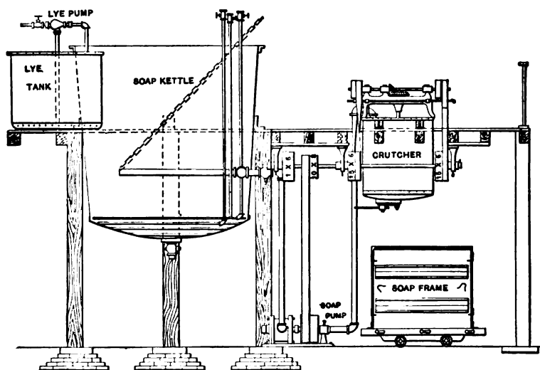
FIG. 44.—Kettle-plant.
