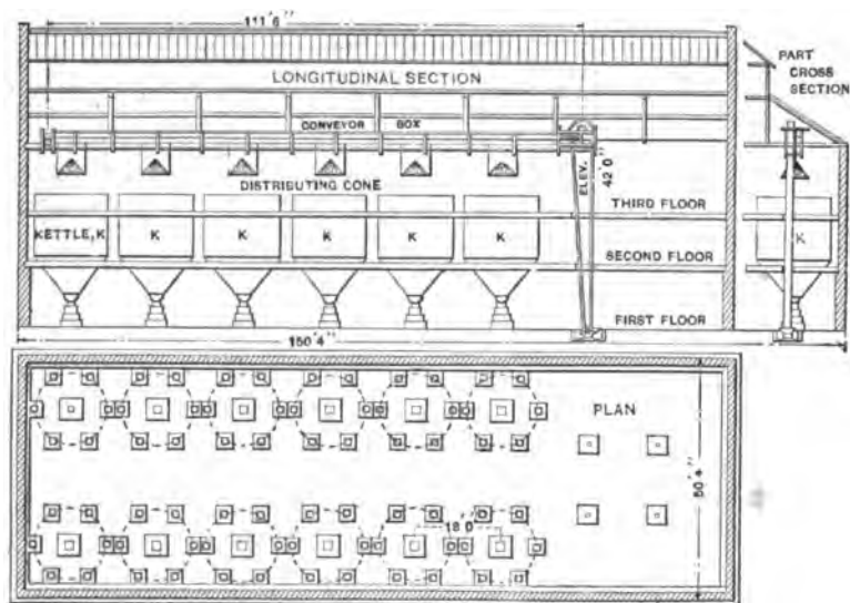
FIG. 48.—Kettle-plant.
