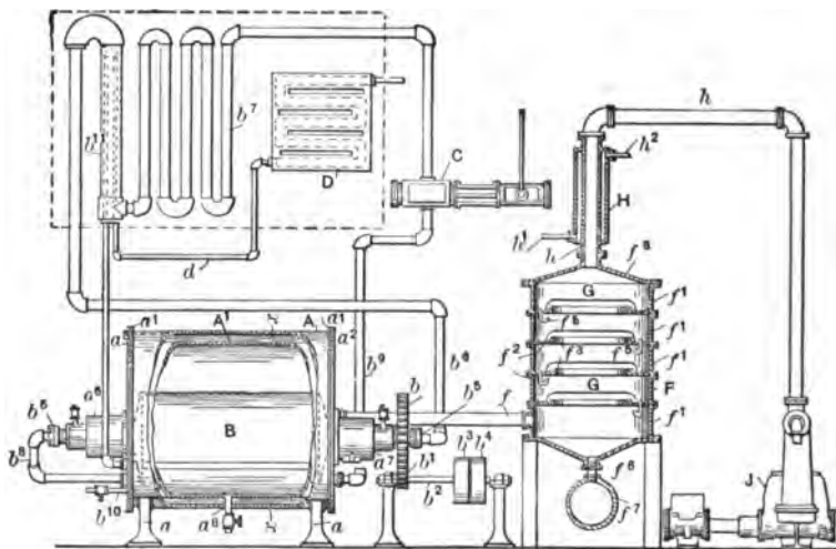
FIG. 222.—Glycerin-still (Joslin System).
