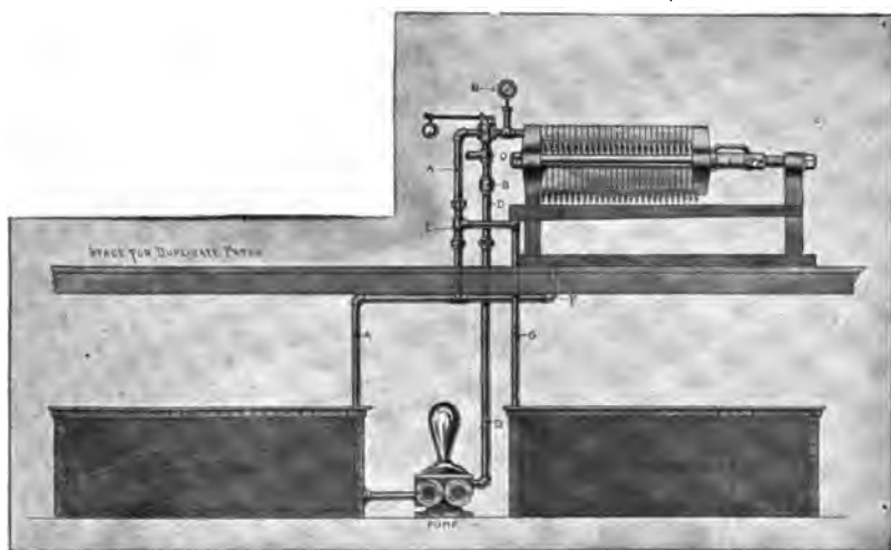
FIG. 35.—Filter-press Plant.
