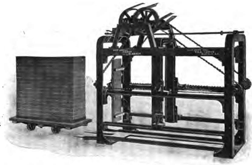
FIG. 84.—Wetherill Power-slabber.
