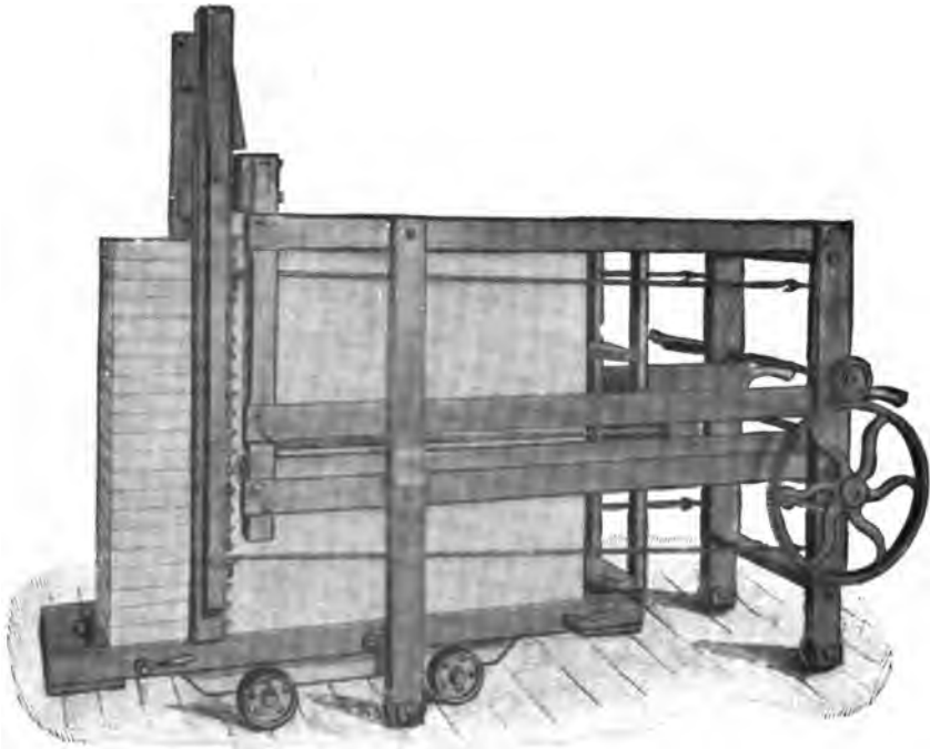
FIG. 82.—Ralston Soap-slabber.
