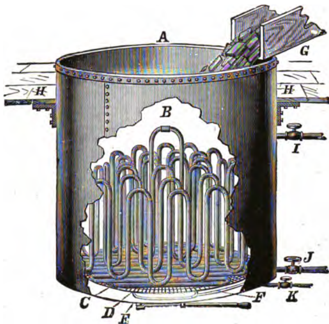
FIG. 94.—Remelter.
