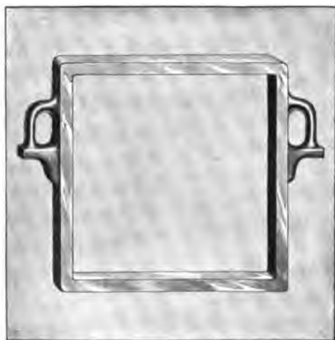
FIG. 33.—Filter-press Frame.
