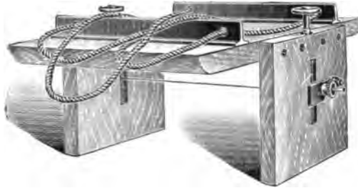
FIG. 81.—Hand Soap-slabber.
