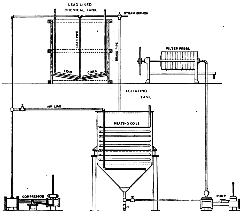
FIG. 30.—Bleaching-plant.
