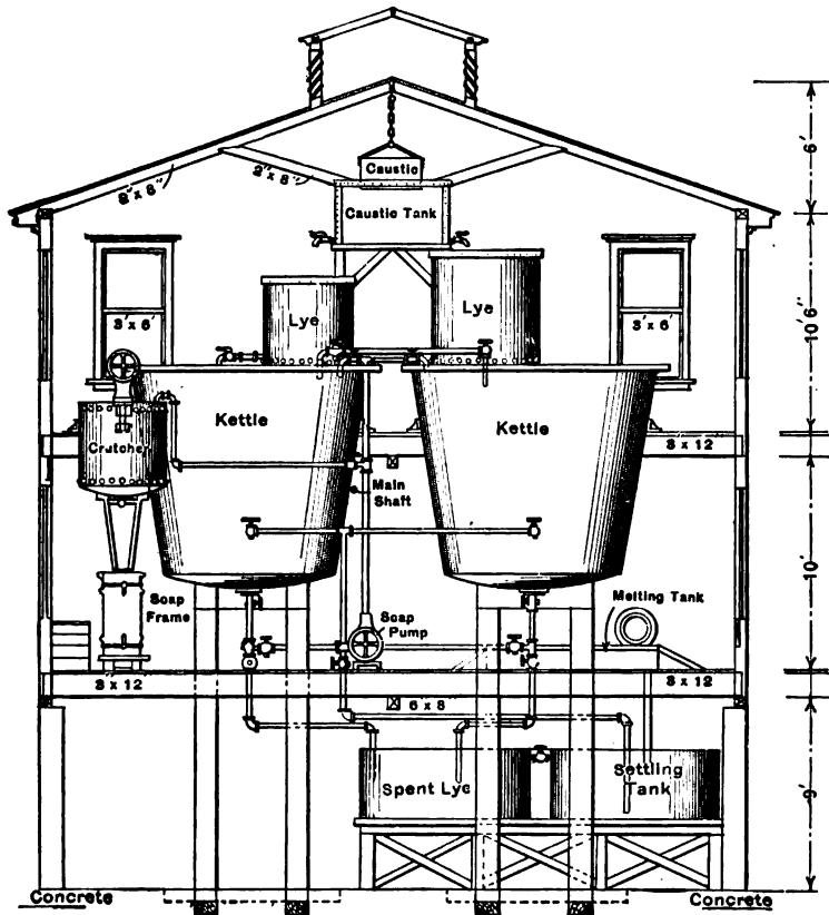
FIG. 45.—Kettle-plant.
