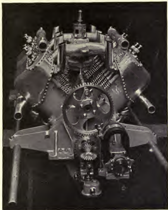
FIG. 69.—Siddeley-Wolseley Motor.
