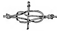
Fig. 171. Double Loop.
