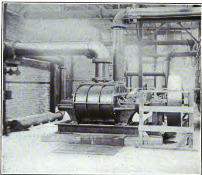
FIG. 71.—Roots blower.
