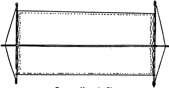
FIG. 192.—Norwegian Rig.
