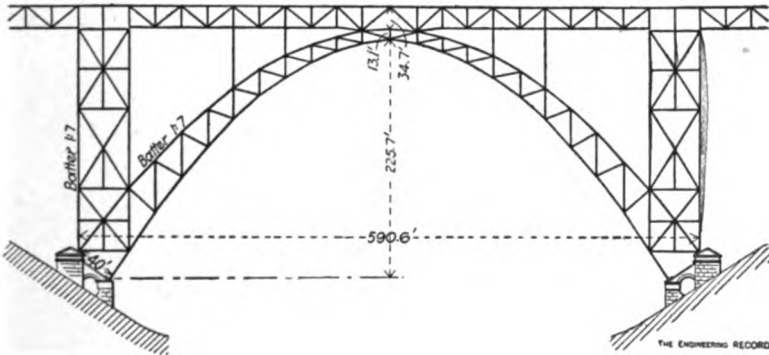
KAISER WILHELM BRIDGE.
