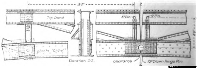
Crown Hinge.
