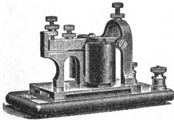
Fig. 12. The Sounder.
