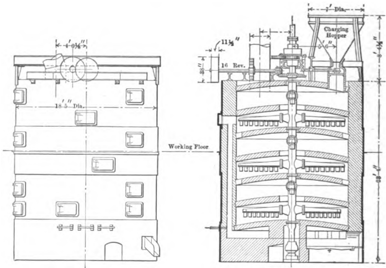
FIG. 14. — McDougall calciner
