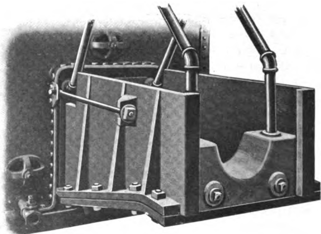
FIG. 33. — Trap-spout
