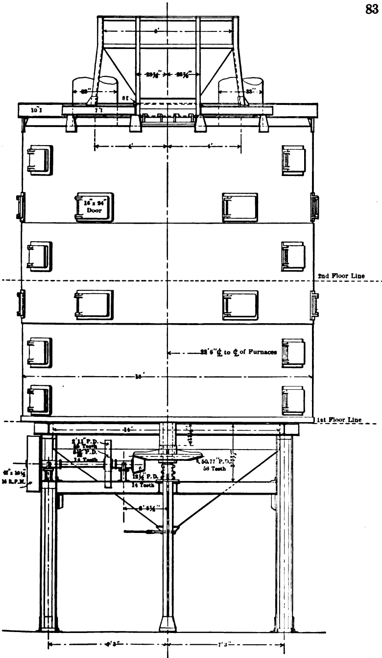
FIG. 15. — McDougall calciner
