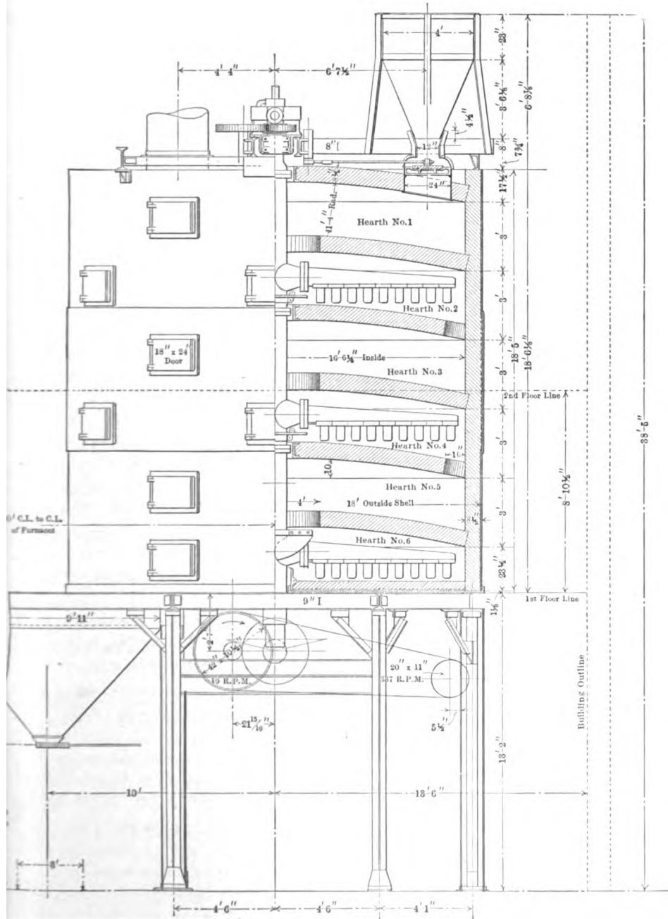
FIG. 16. — McDougall calciner
