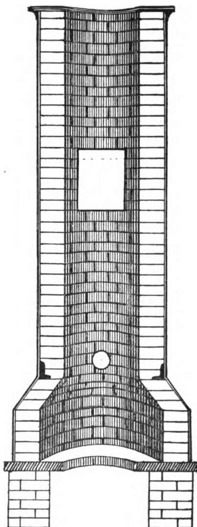
RESERVOIR CUPOLA.
