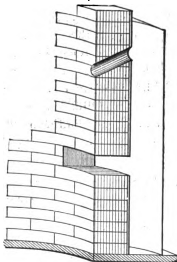
COLLIAU TUYERE.
