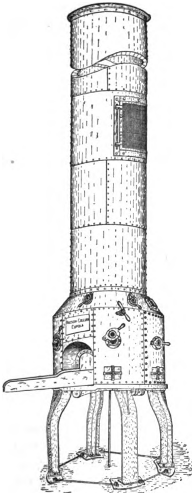
PAXSON HOT BLAST CALLIAU CUPOLA.
