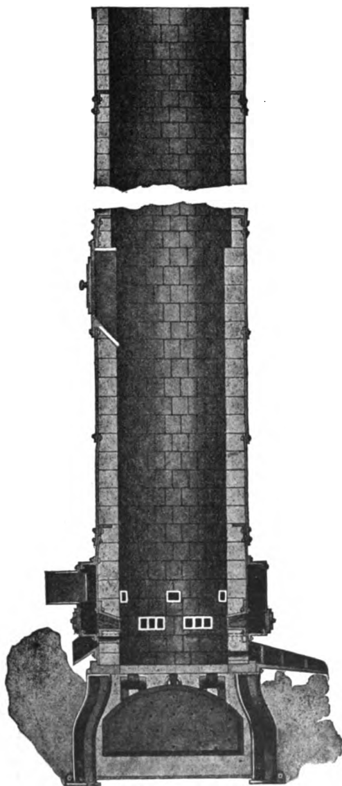
THE NEWTEN CUPOLA.
