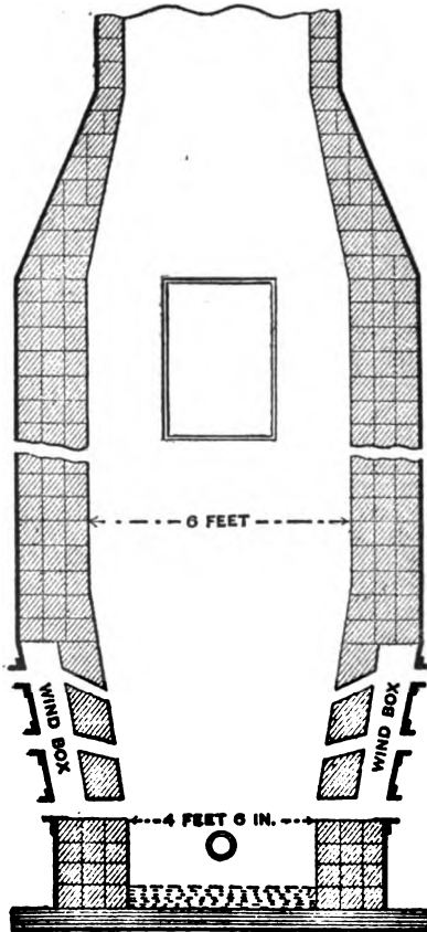
JUMBO CUPOLA.
