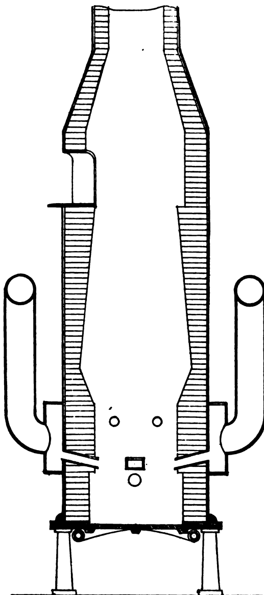
VOISIN'S CUPOLA.
