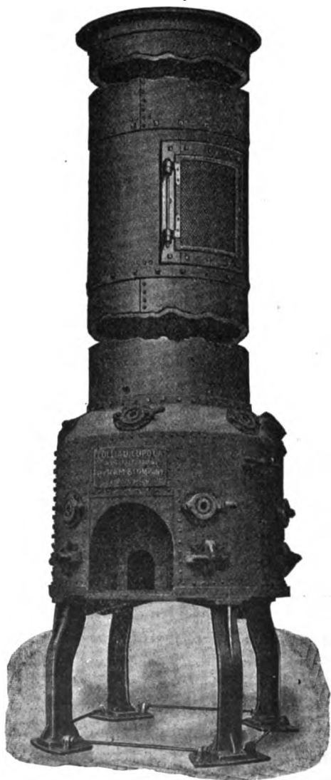
COLLIAU CUPOLA.
