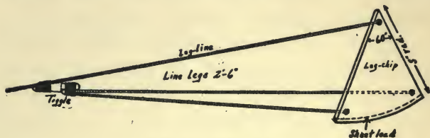
FIG. 1.—Chip Log.
