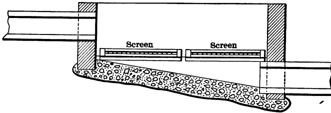
LONGITUDINAL-SECTION
