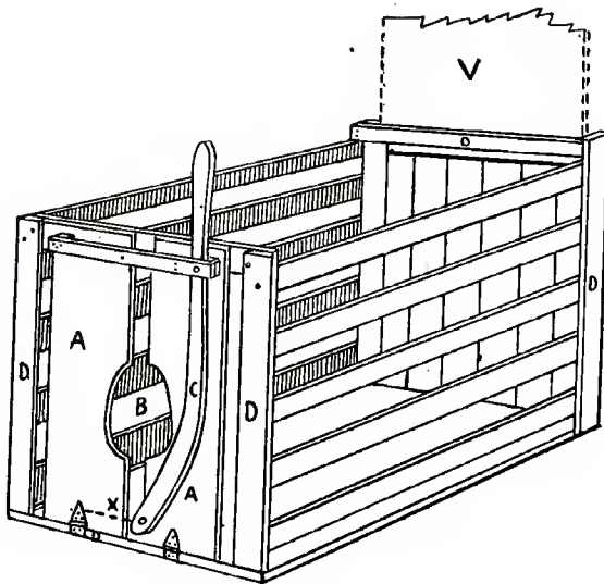
Fig. 317. Hog Trap.
