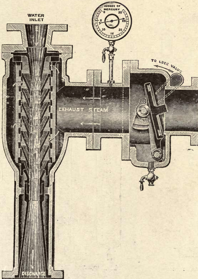
Fig. 146.—Ledward Ejector Condenser.
