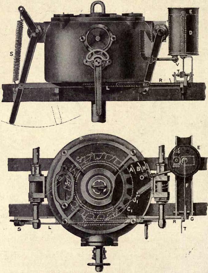
Fig. 330.—“ Watson-Laidlaw ” Impulse Motor for “ Weston ” Centrifugal Machines.
