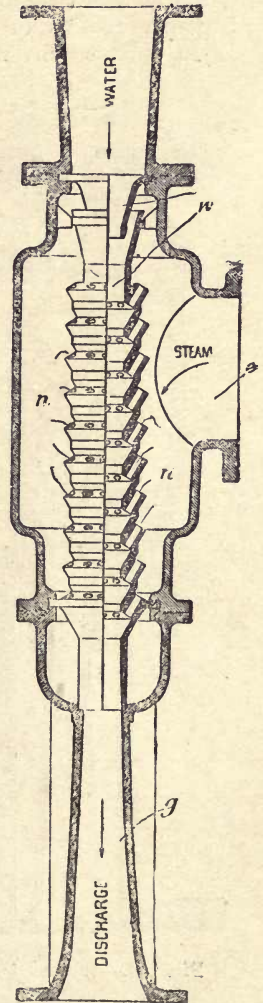
Fig. 147.—Körting Ejector Condenser.
