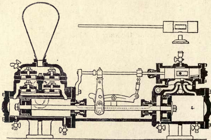
Fig. 87.—Blake-Knowles Simplex Pump.
