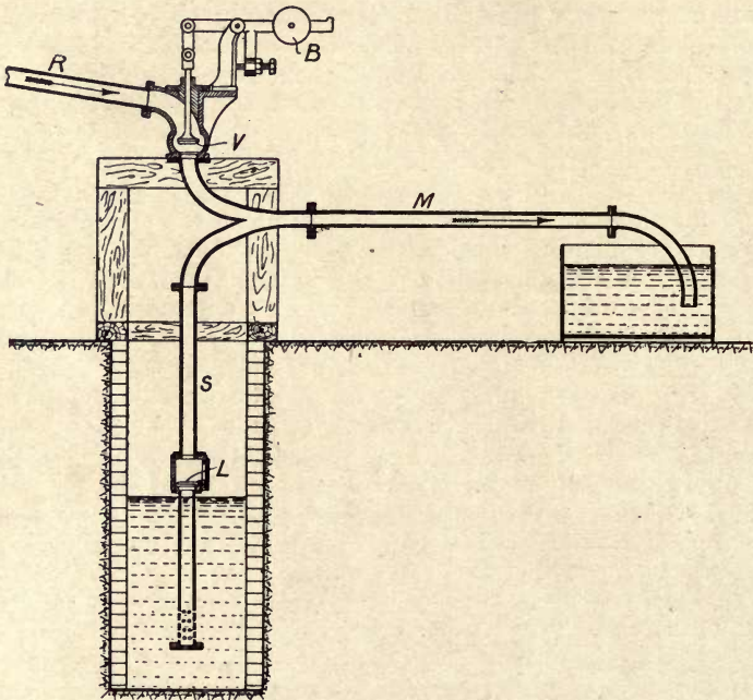
Fig. 180. Leblanc Siphon Ram.
