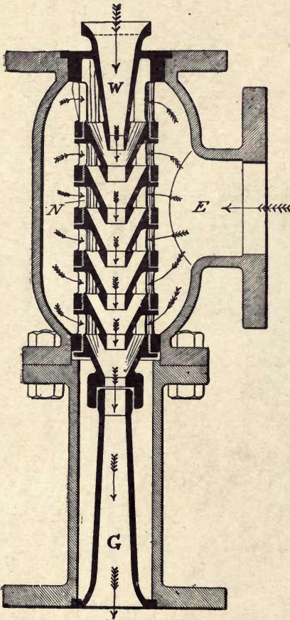
Fig. 148.—White Ejector Condenser.
