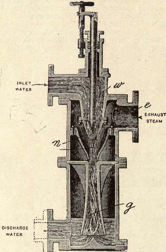
Fig. 145.—Morton's Ejector Condenser.
