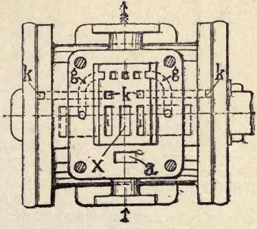
Fig. 106.—Valve Gear Details of Voit Pump.
