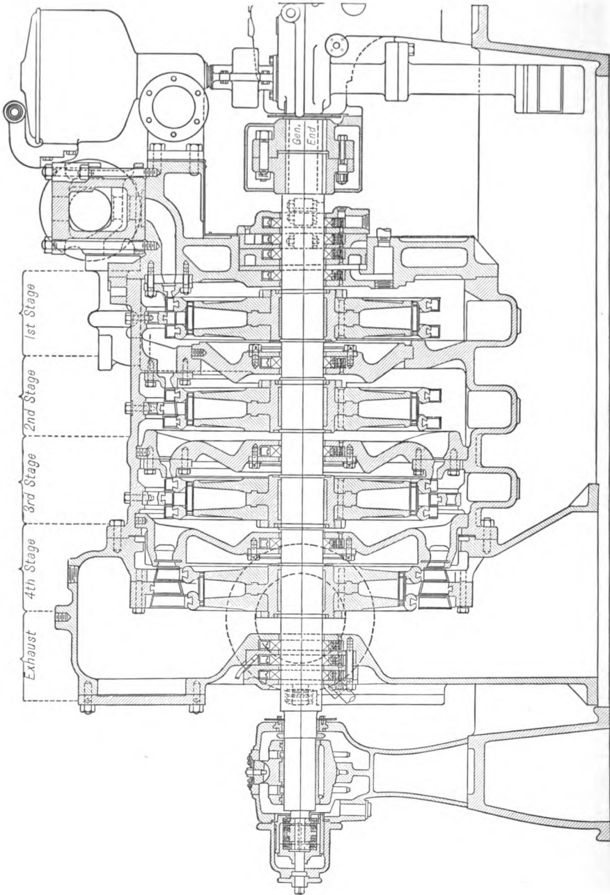
FIG. 172. Curtis Turbine.
