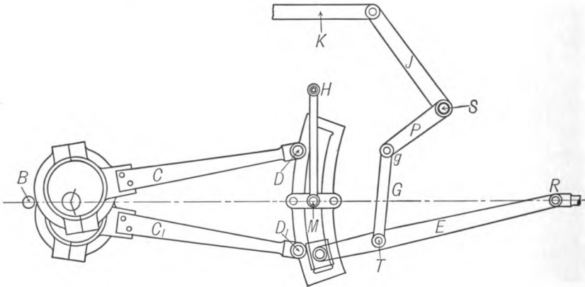
FIG. 148. Gooch Link.
