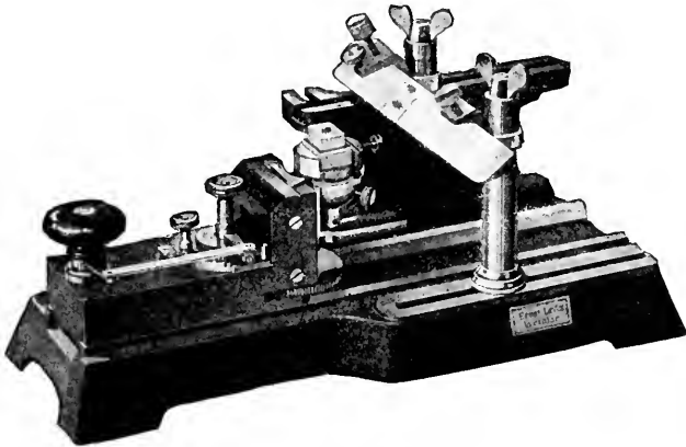
FIG. 36.—Base Sledge Microtome
