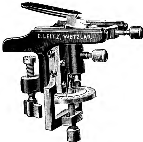
FIG. 35.—Hand Table Microtome
