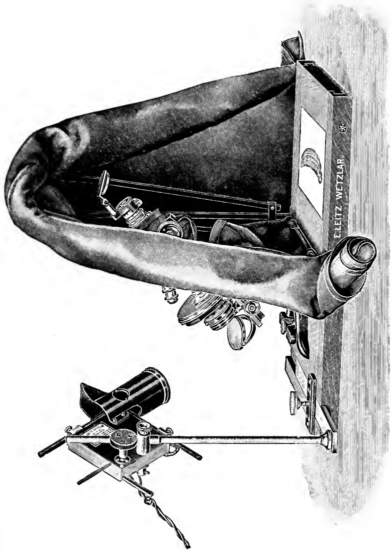
FIG. 28.—Drawing Apparatus
