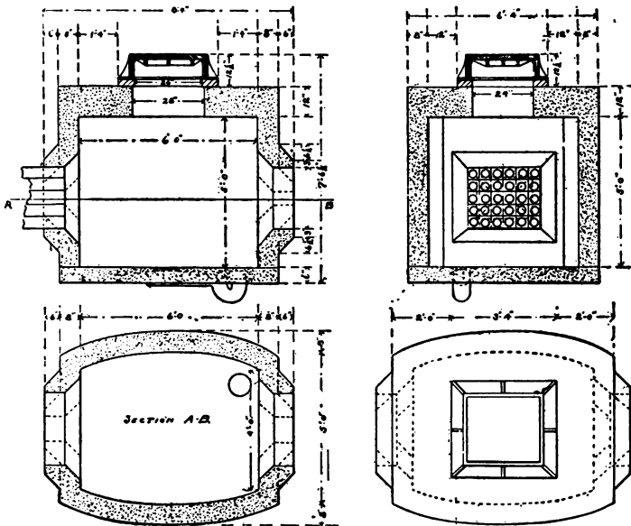
Fig. 29. Standard Manhole.
