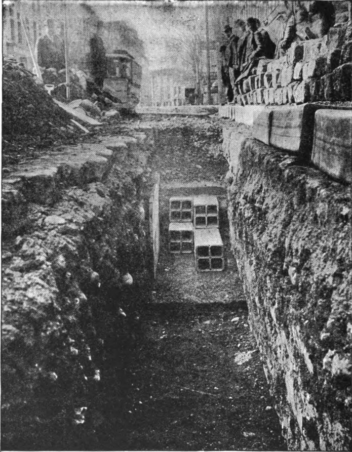
Fig. 17. Multiple Duct Conduit.
