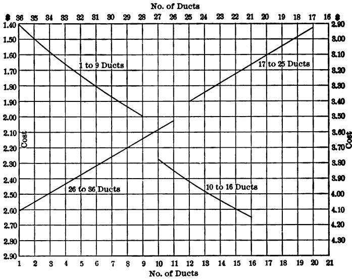
Fig. 54. Cost per Conduit Foot; Average.
