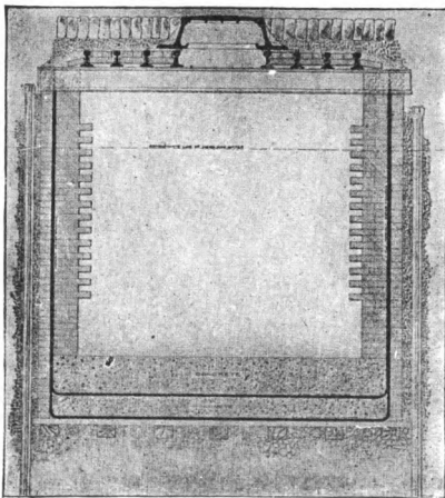
Fig. 39. Waterproof Manhole.
