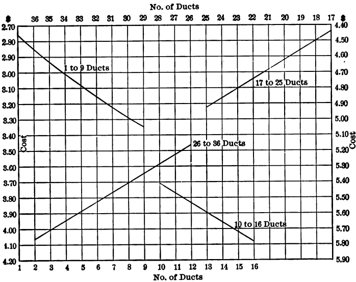
Fig. 55. Cost per Conduit Foot; Average.
