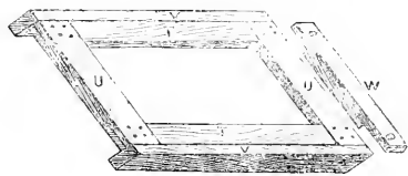
Fig. 14.—Frame-fastener.
