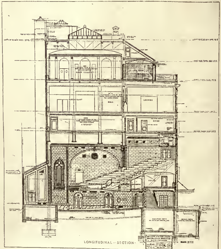
LONGITUDINAL SECTION
