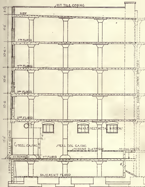
LONGITUDINAL SECTION
