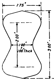
FIG. 88.—Standard Briquette.
