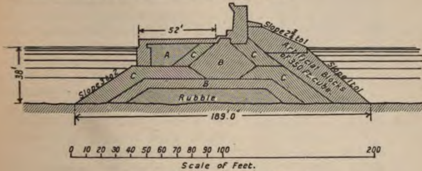
FIG. 118.—Digue de la Joliette, Marseilles.
