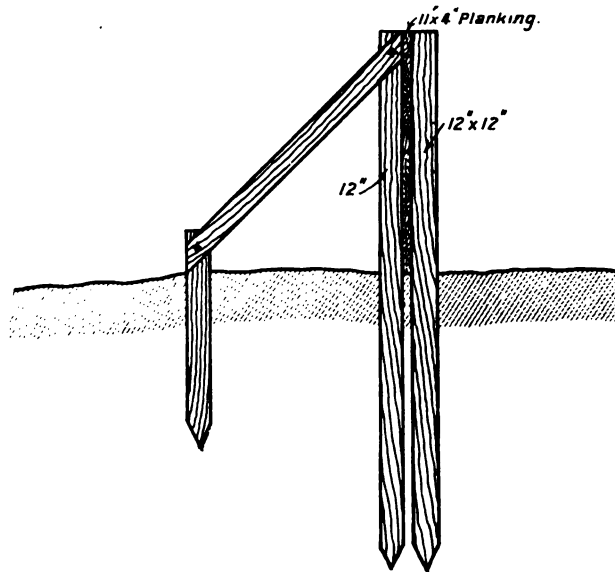
FIG. 211.—Timber Groyne.
