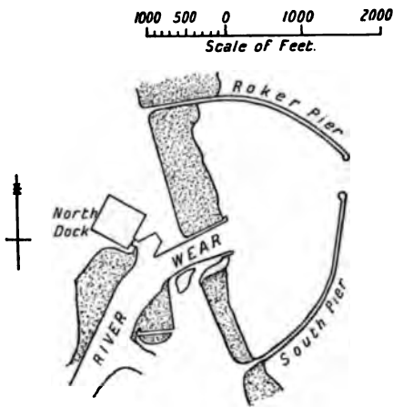
FIG. 4.—Sunderland Harbour.
