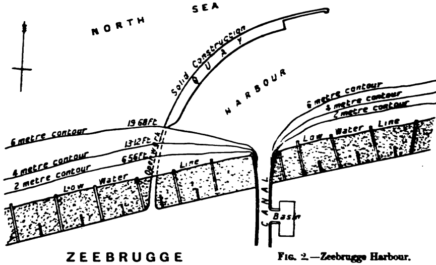
FIG. 2.—Zeebrugge Harbour.
