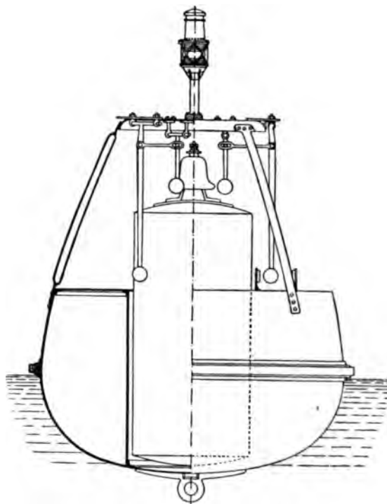
FIG. 246. — Bell-buoy.
