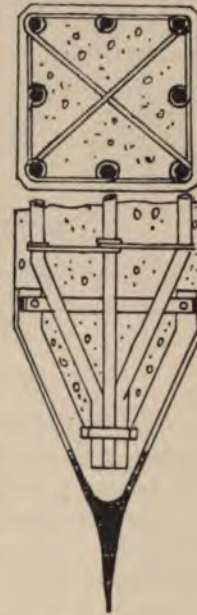
FIG. 66.— Hennebique Pile.
